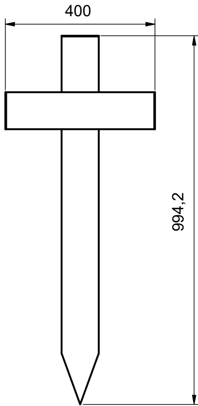
Vorderansicht
